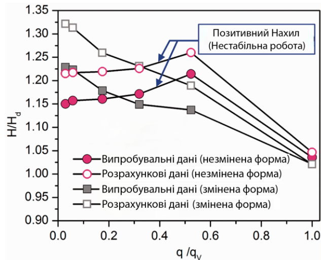
Рисунок 1. Криві продуктивності насосів із різними формами лопатей отримані експериментально і чисельно
